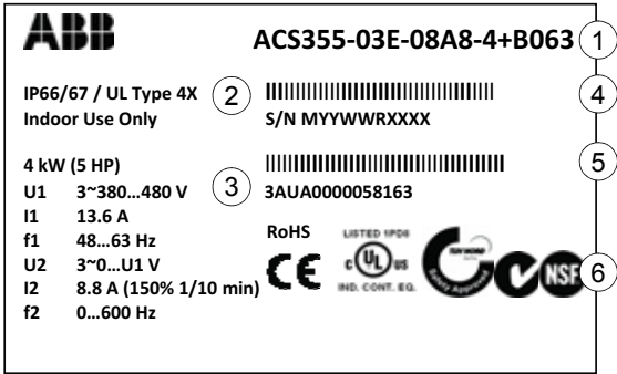
Plaque signalétique
