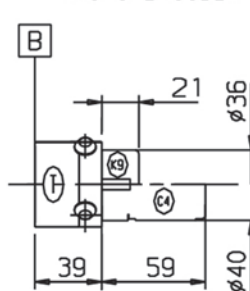
TACHO+ENCODER
