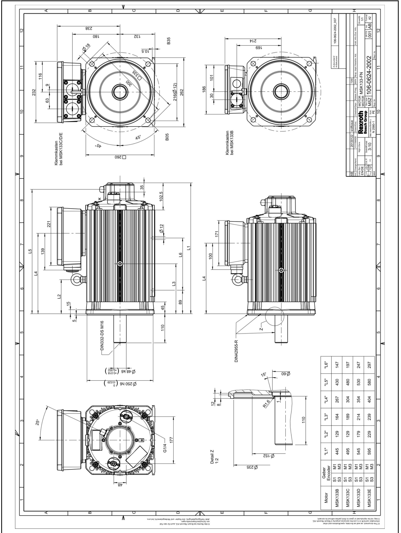
Fig. 5-36: MSK133-_-FN
