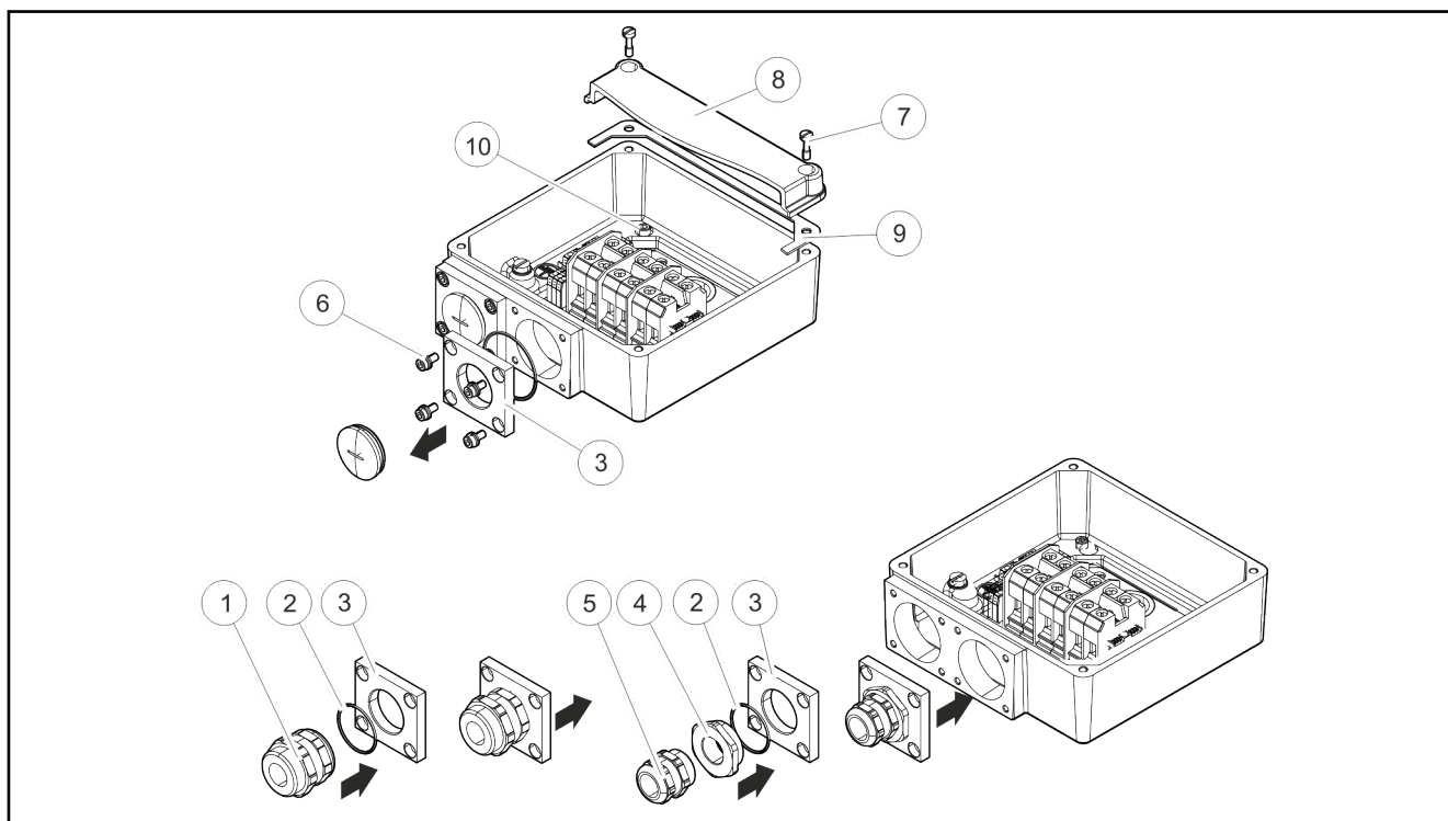
Fig. 12-1: MSK133
