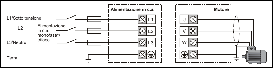
Figura 6-1 Connessioni dei terminali di potenza
