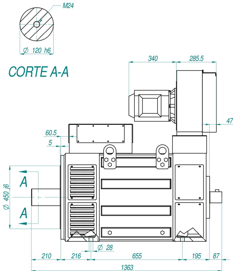
MOTOR MAC QT 315 M DIMENSIONS
