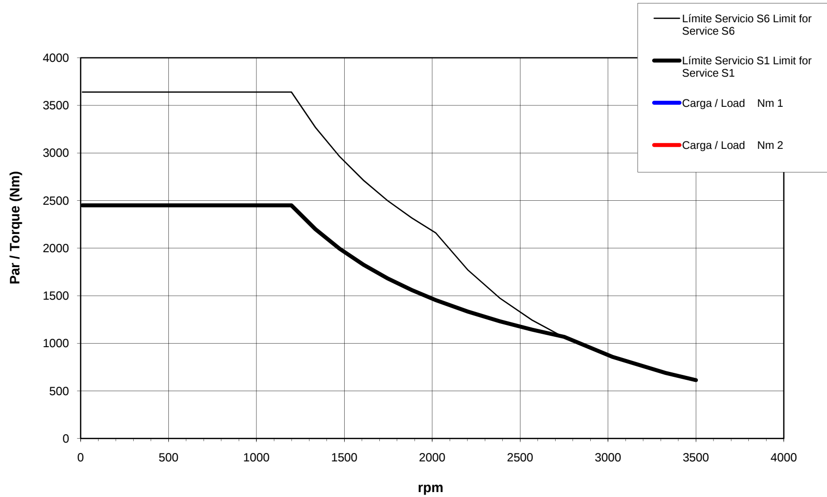
Curva de Par / Torque Diagram
