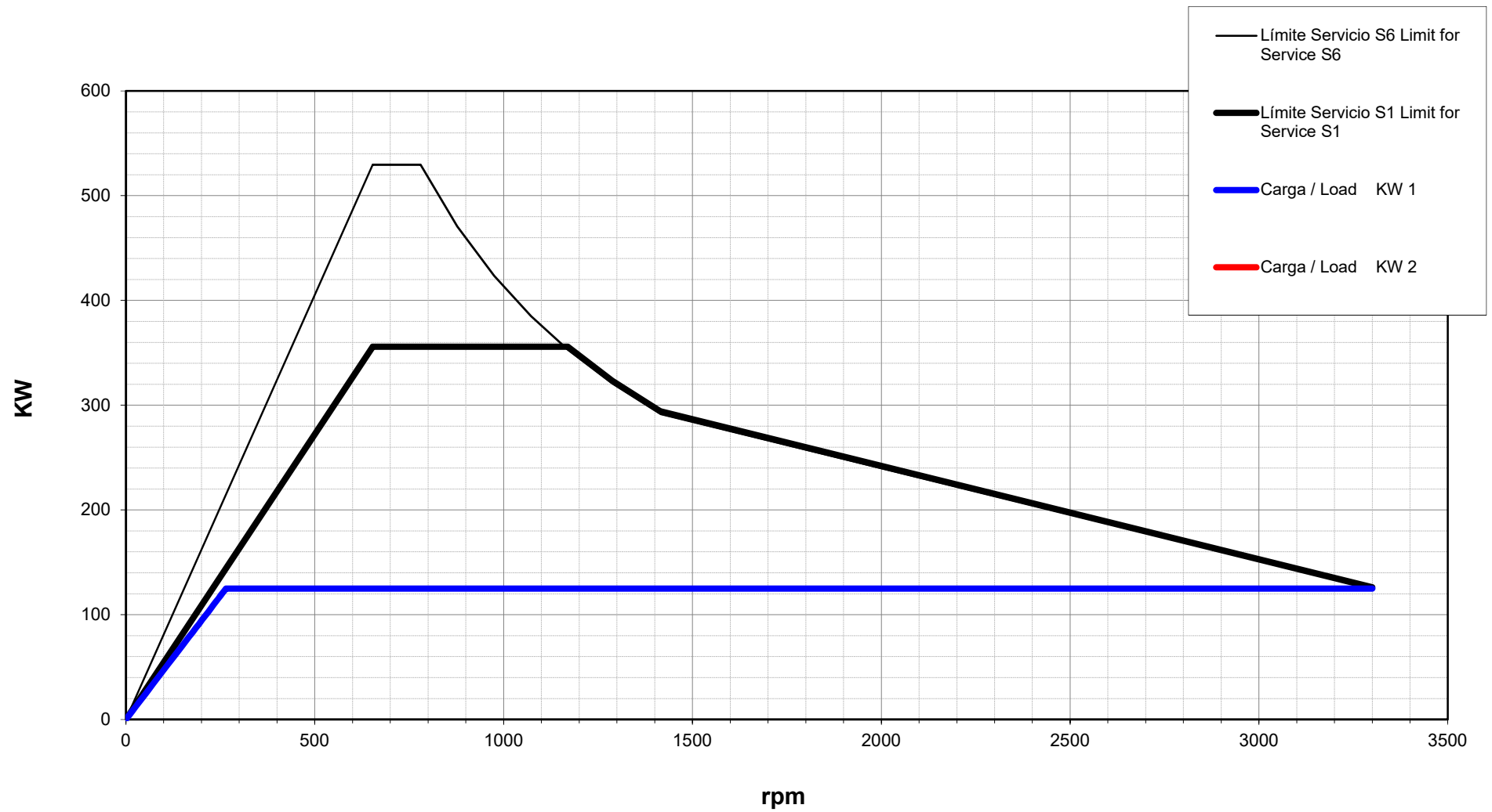
Curva de Potencia / Power Diagram
