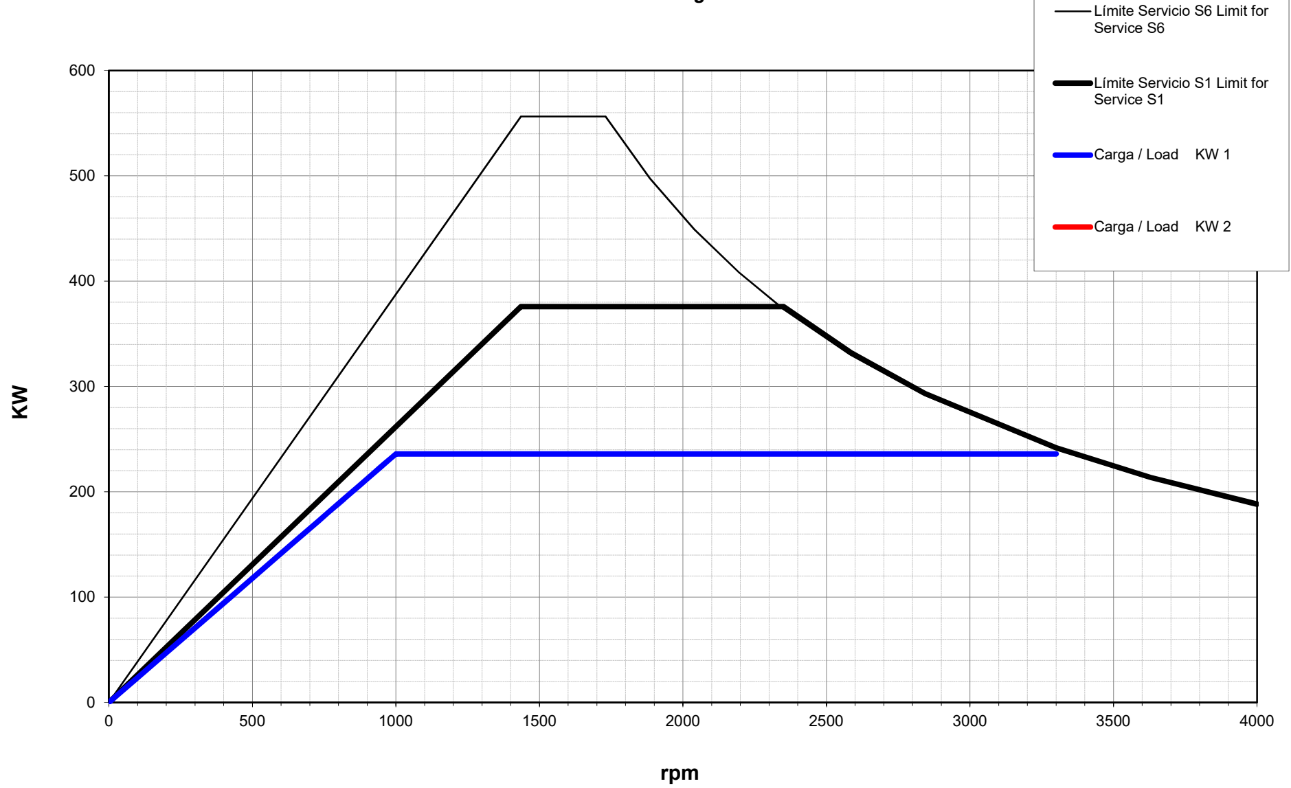
Curva de Potencia / Power Diagram
