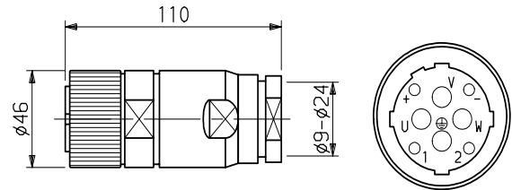
PLUG 220065R3610/3611
