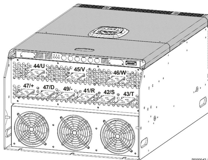
Figura 11: Barre di collegamento S41-S42-S51-S52
