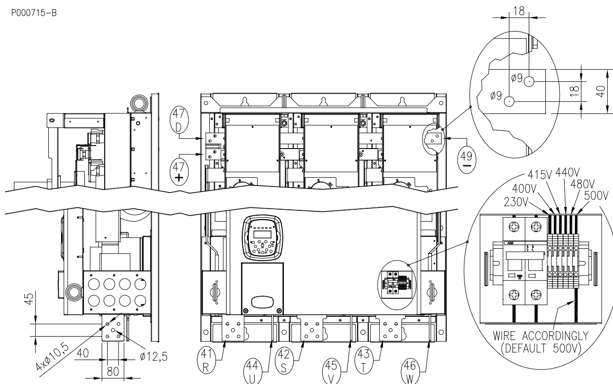
Figura 12: Barre di collegamento S60
