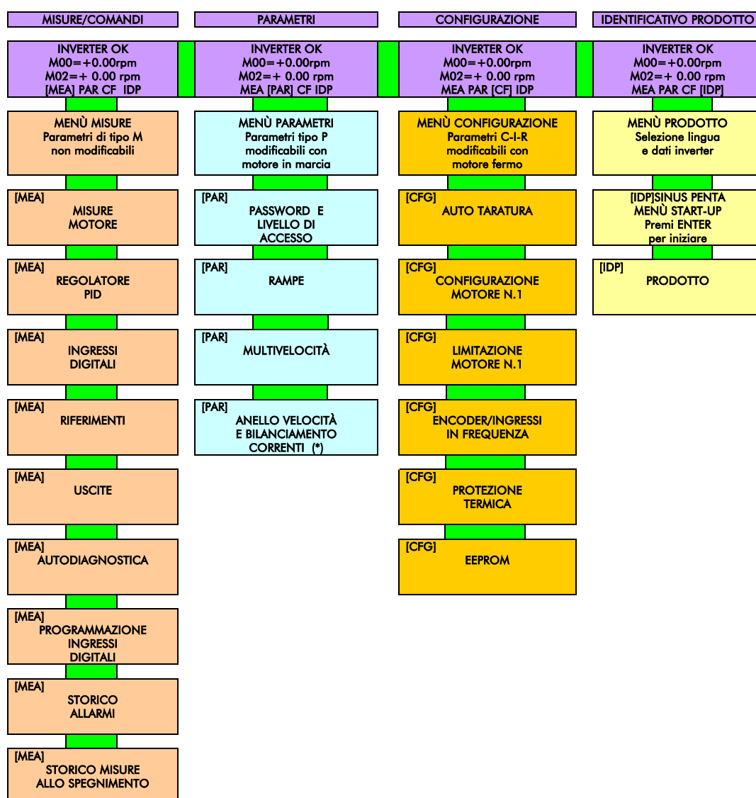
Figura 16: Struttura ad albero dei menù
