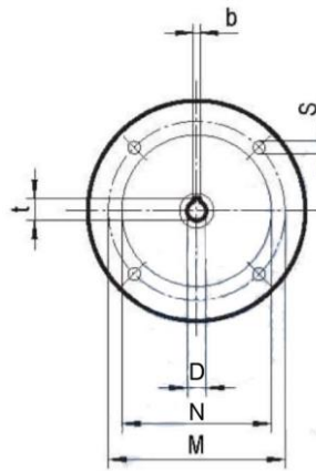
Input Flange
