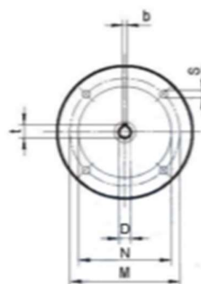
Input Flange
