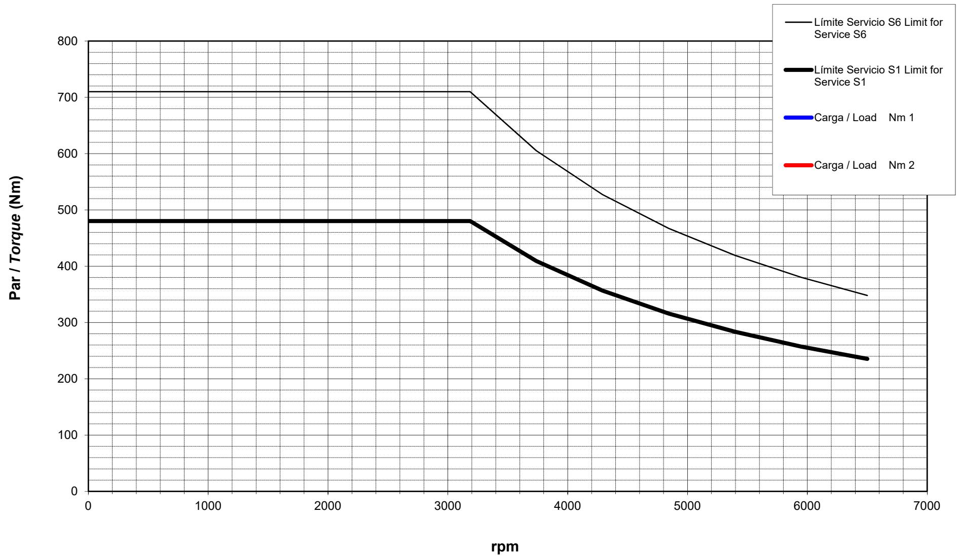
Curva de Par / Torque Diagram
