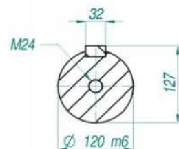
CORTE A-A
