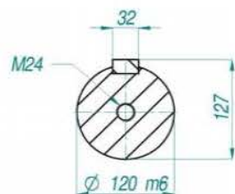
CORTE A-A
