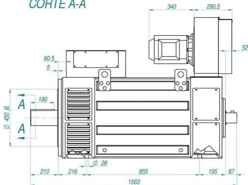
CORTE A-A
