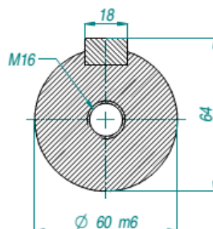
CORTE A-A
