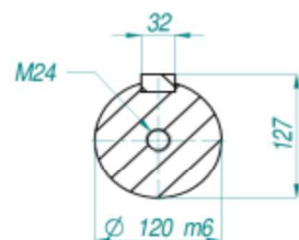
CORTE A-A
