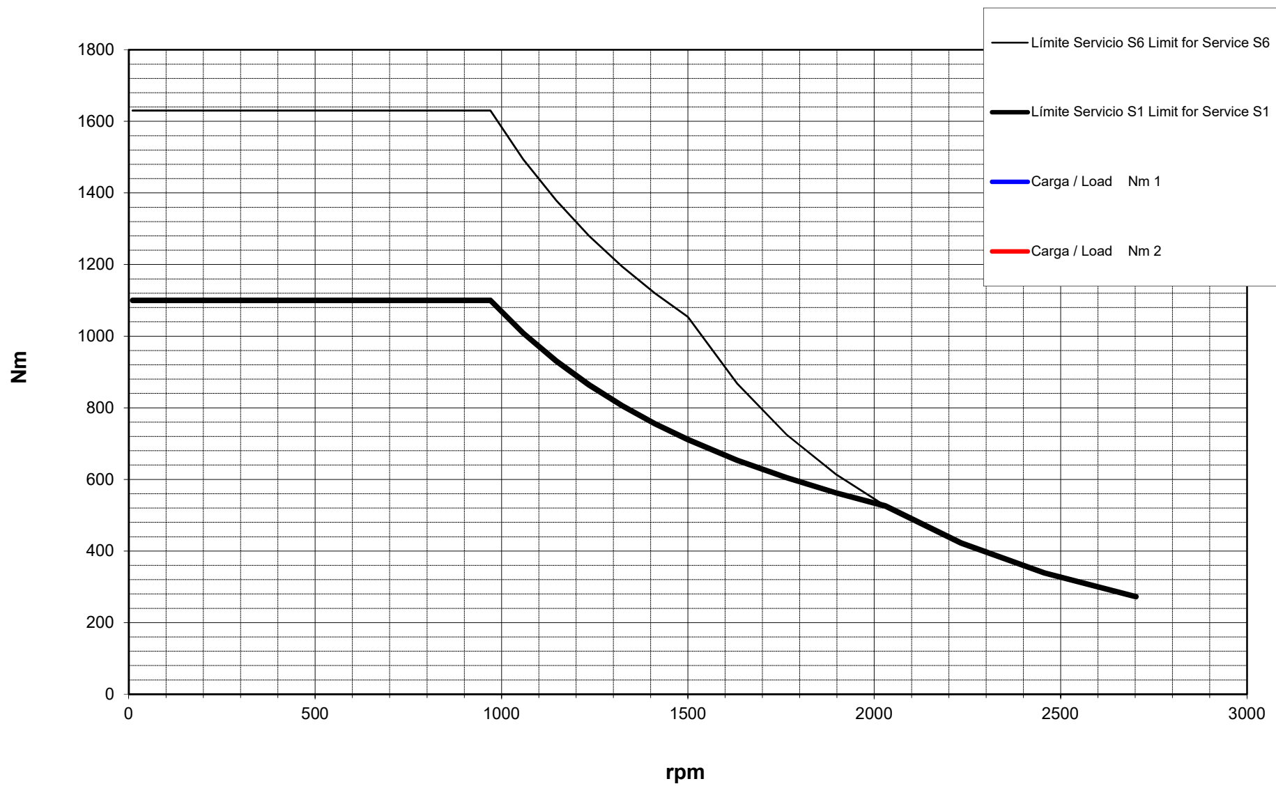
Curva de Par / Torque Diagram
