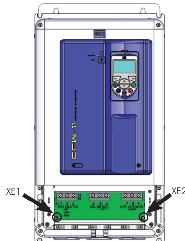
(d) Frame size D - IP2X or Nema1
