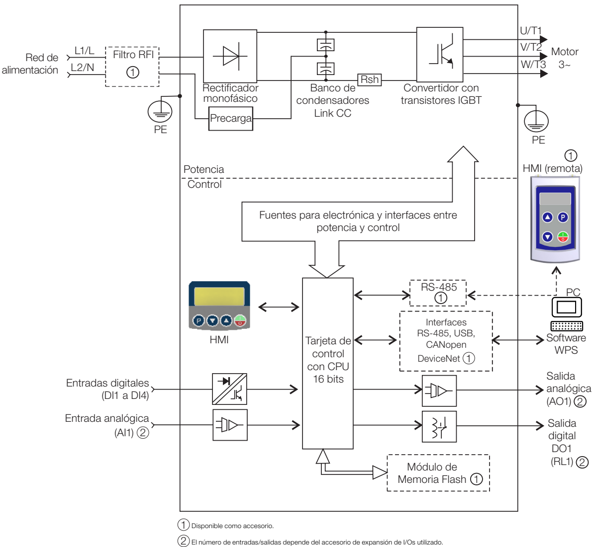
Figura 2.2: Diagrama de bloques del CFW100 para el tamaño 110 V
