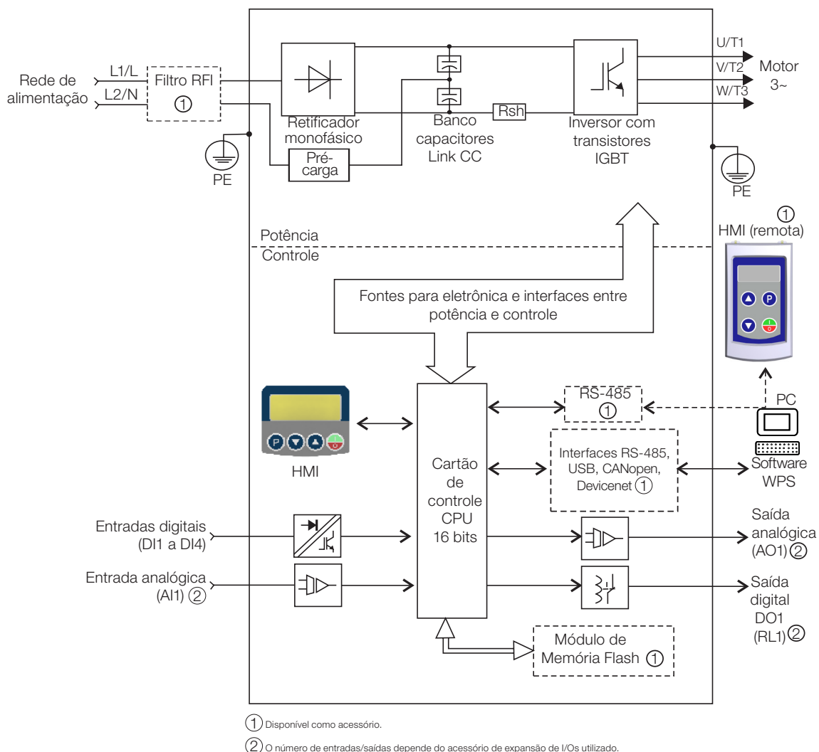
Figura 2.2: Blocodigrama do CFW100 para modelos 110 V
