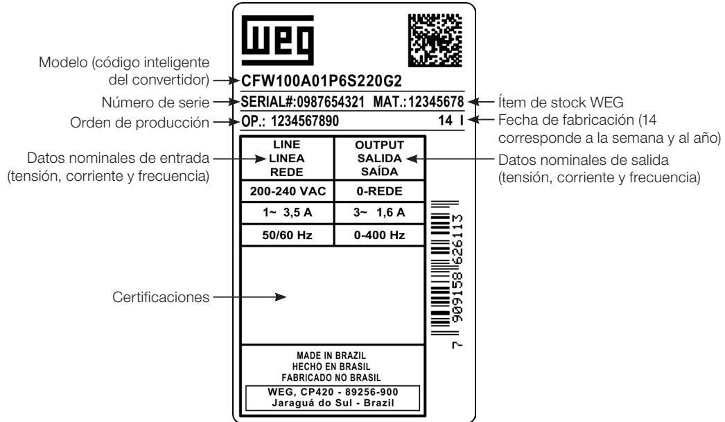
Etiqueta Lateral del CFW100
