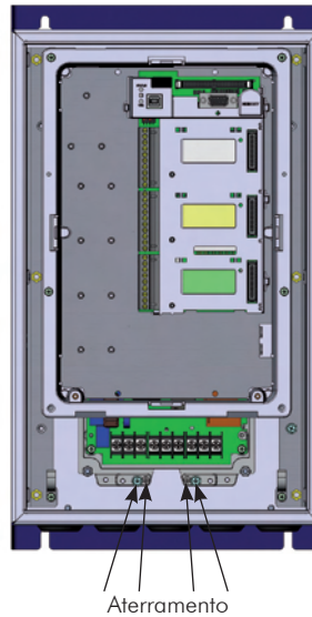
Figura 3 - Aterramento do produto
