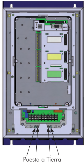
Figura 3 - Puntos de puesta a tierra del producto
