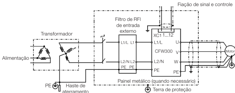
Figura 3.5: Conexão do filtro supressor de RFI - condição geral
