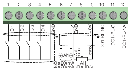
(a) Configuración NPN
