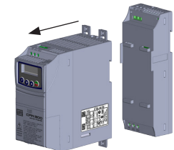
(b) Fit the filter set on the CFW300 base (b) Encaje el conjunto filtro en la base del CFW300 (b) Encaixe o conjunto filtro na base do CFW300
