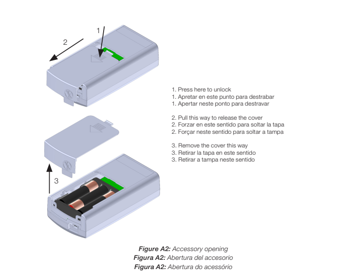
Figure A2: Accessory opening Figura A2: Abertura del accesorio Figura A2: Abertura do acessório
