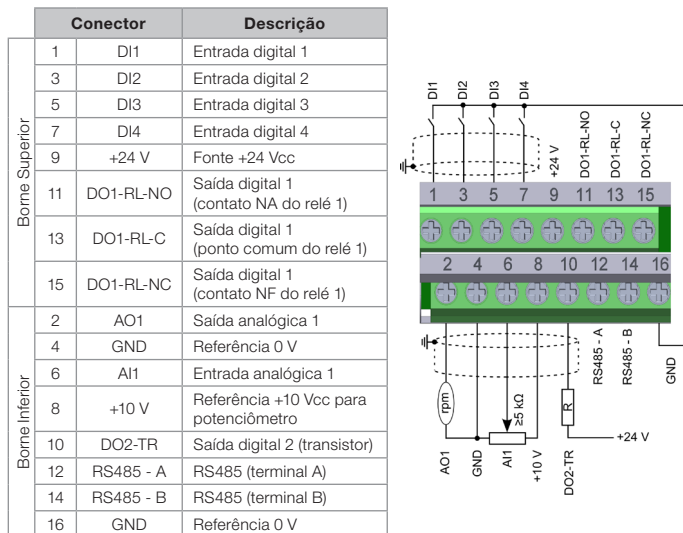
Figura 1: Sinais do conector de controle
