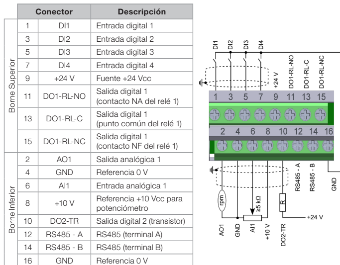
Figura 1: Señales del conector de control
