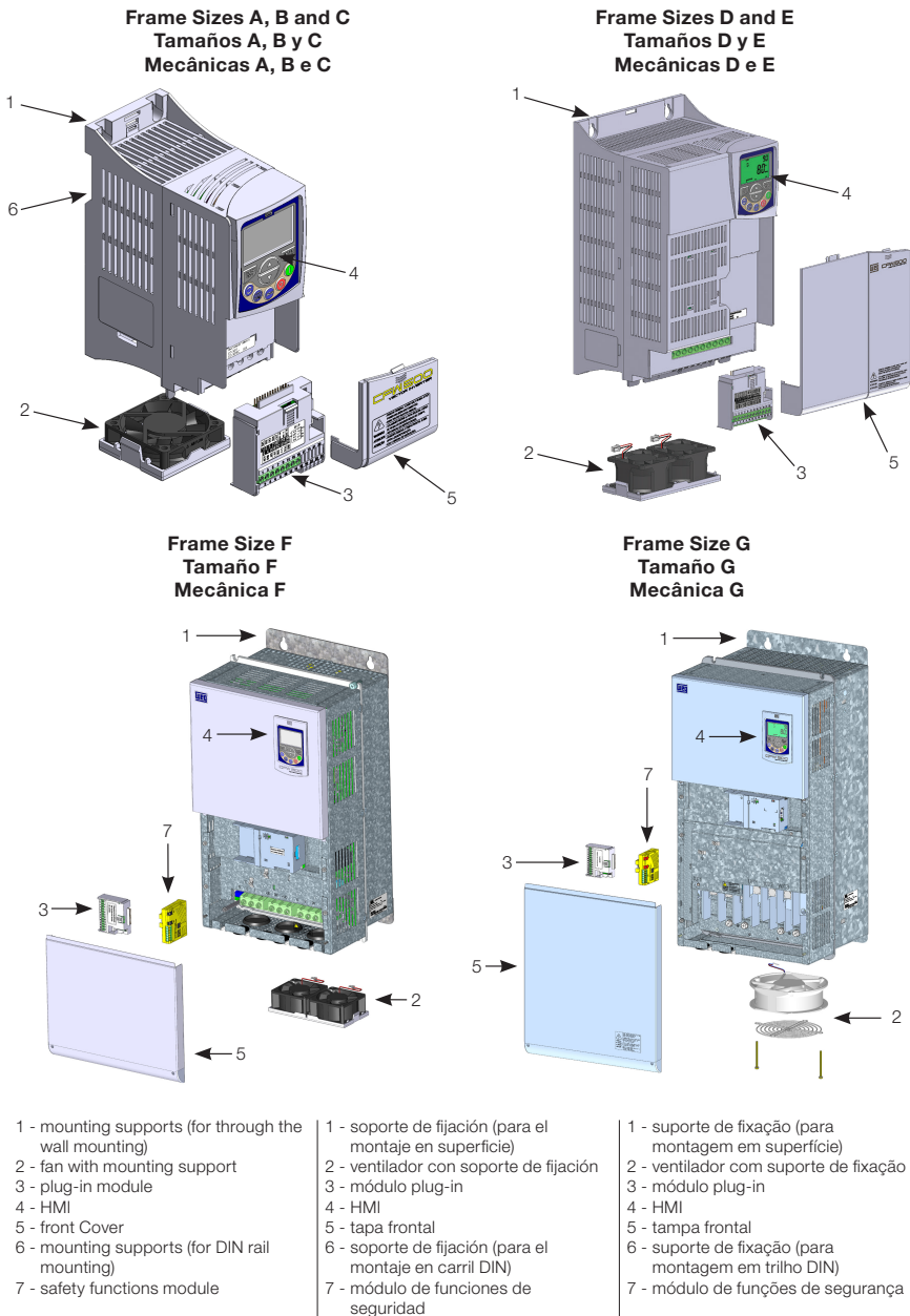
Figure A.1: Main components of the CFW500 Figura A.1: Principales componentes del CFW500 Figura A.1: Componentes principais do CFW500
