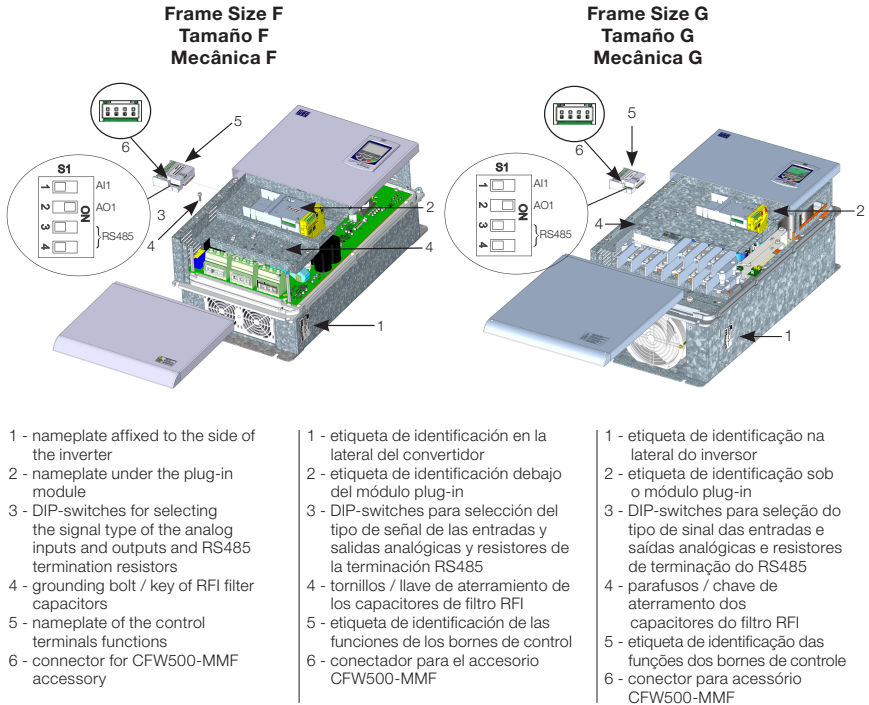
Figure A.2: Location of the nameplates and DIP-switches Figura A.2: Localización de las etiquetas de identificación y DIP-switches Figura A.2: Localização das etiquetas e DIP-switches
