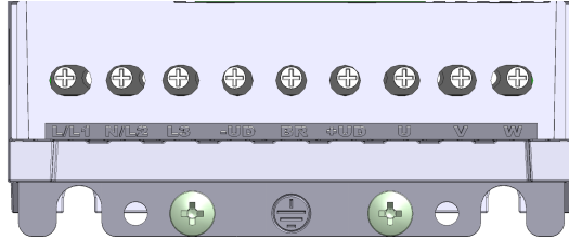
Frame Size B / Tamaño B / Mecânica B
