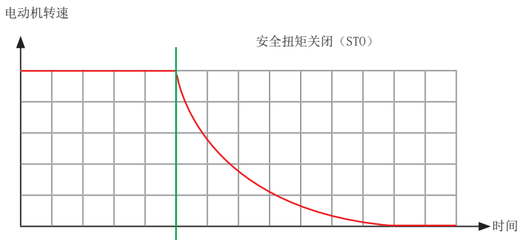
图1.1 STO操作
