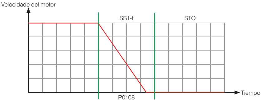
Figura 1.2: Comportamiento SS1-t
