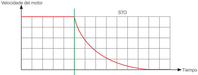
Figura 1.1: Comportamiento STO
