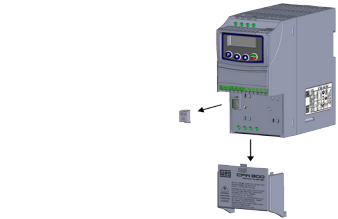
(a) Removal of the accessory and connection protection covers (XC4) from the IO expansion connector (a) Remoción de las tapas de accesorios y de protección de la conexión (XC4) de la expansión de IO's (a) Remoção das tampas de acessórios e de proteção da conexão (XC4) da expansão de IO's
