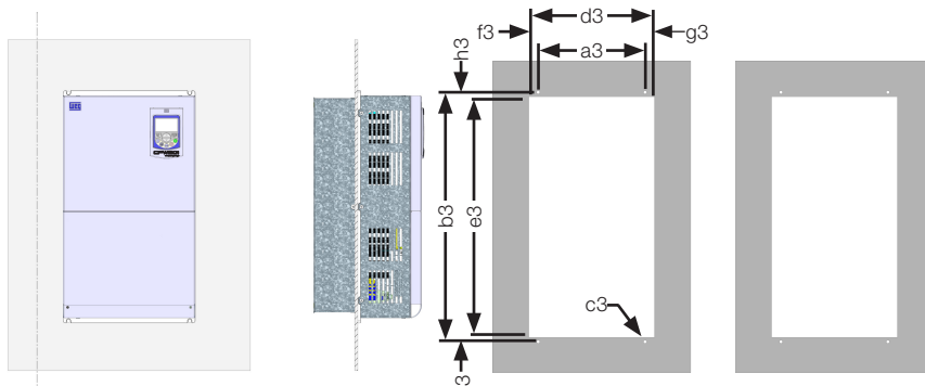
(c) Flange mounting - standard inverter (Only frame sizes F, G) (c) Montaje en flange - convertidor estándar (Solamente tamaños F, G) (c) Montagem em flange - inversor padrão (Somente mecânicas F, G)
