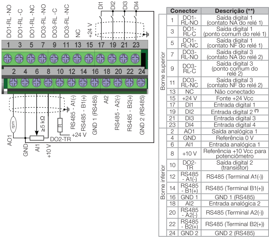
Figura 3.4: Sinais do conector do módulo plug-in CFW500-CRS485-B
