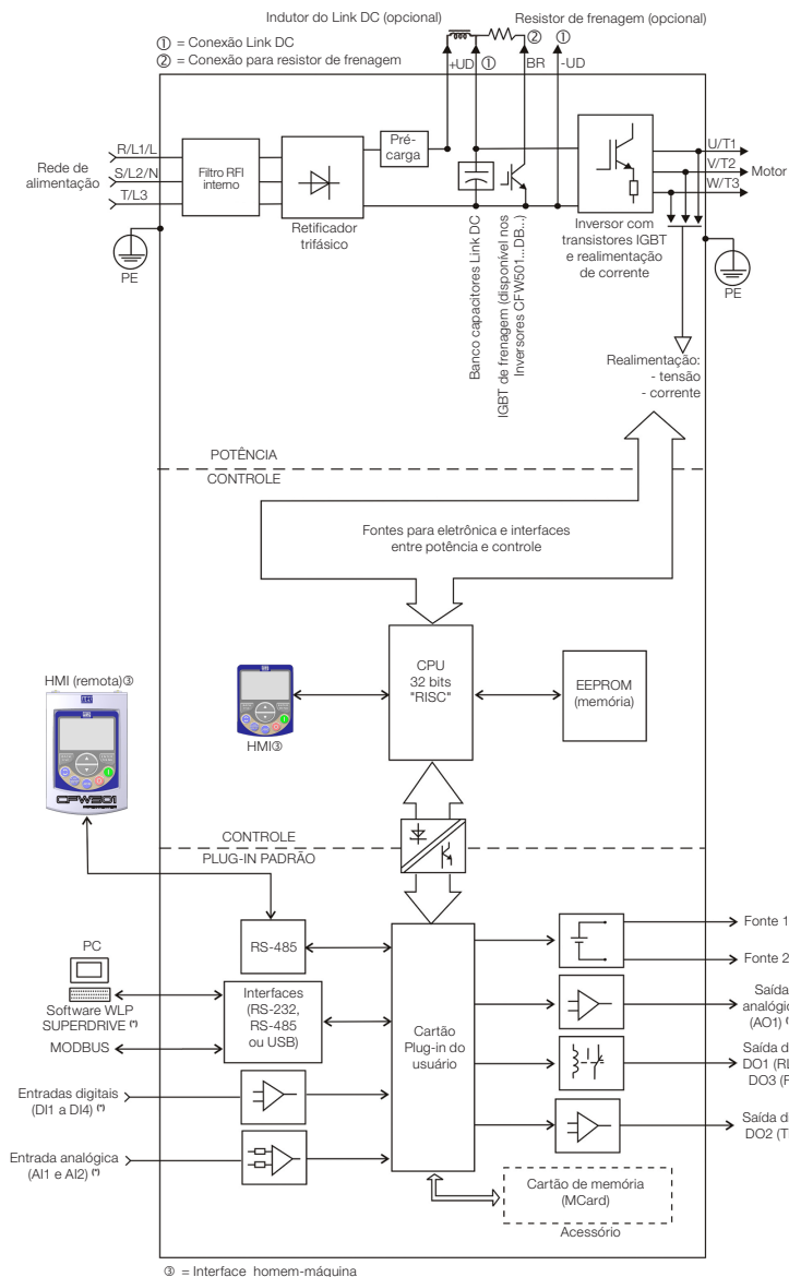
Figura 2.2: Blocodiagrama do CFW501 para mecânicas D e E
