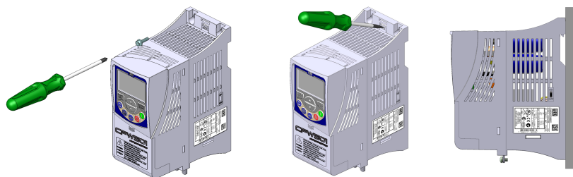
(a) Surface mounting (a) Montaje en superficie (a) Montagem em superfície (b) DIN rail mounting (Only frame sizes A, B, C) (b) Montaje en riel DIN (Solamente tamaños A, B, C) (b) Montagem em trilho DIN (Somente mecânicas A, B, C)
